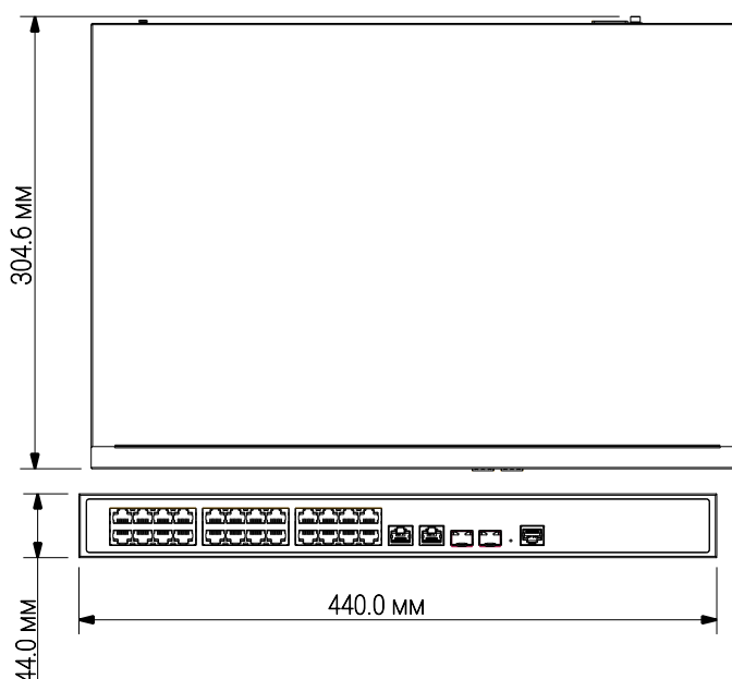
Рисунок 5.1 – Габаритные размеры
