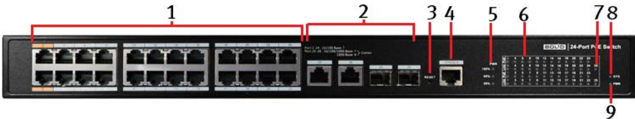
Рисунок 4.1 – Передняя панель конструкции
