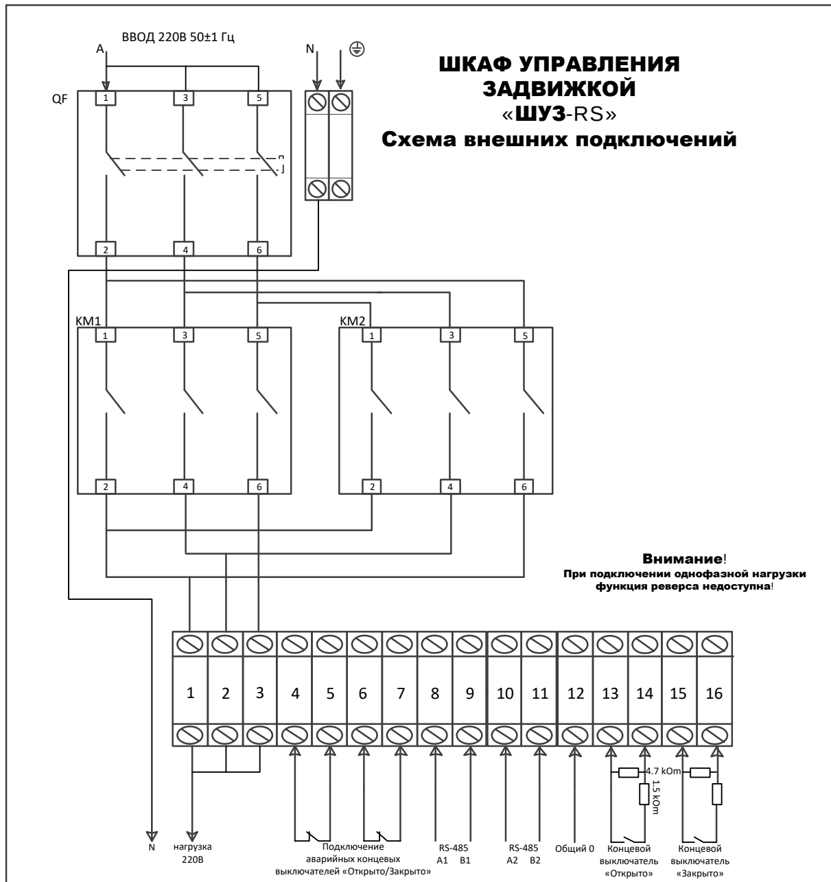
Рисунок 3. Схема подключения блока с однофазной нагрузкой
