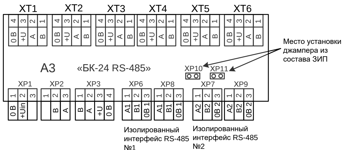
Рис.3 Схематичное изображение разъемов на плате БК-24 RS485, крышка открыта.
