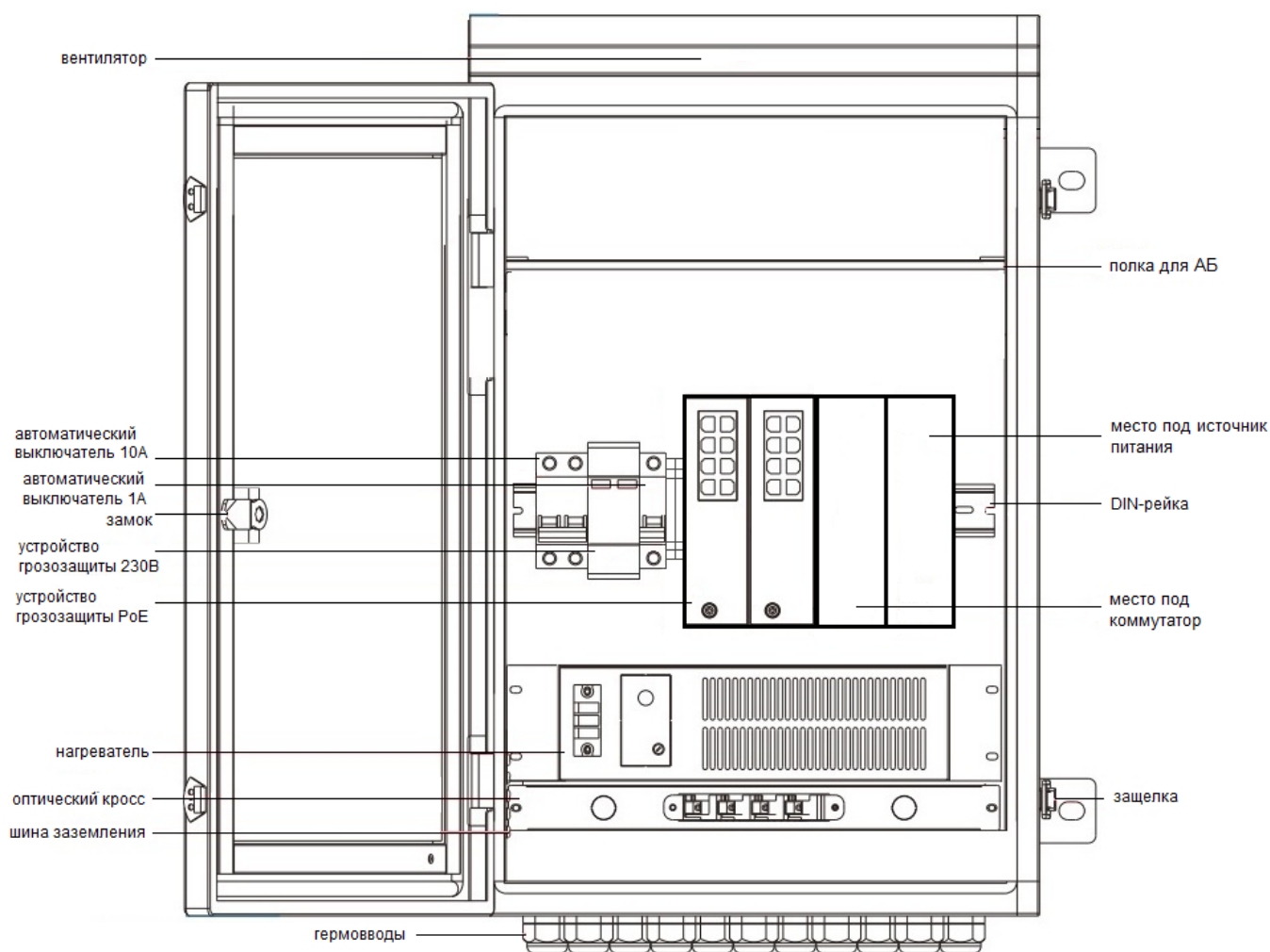
Рисунок 1. Общий вид ШКУ-01
