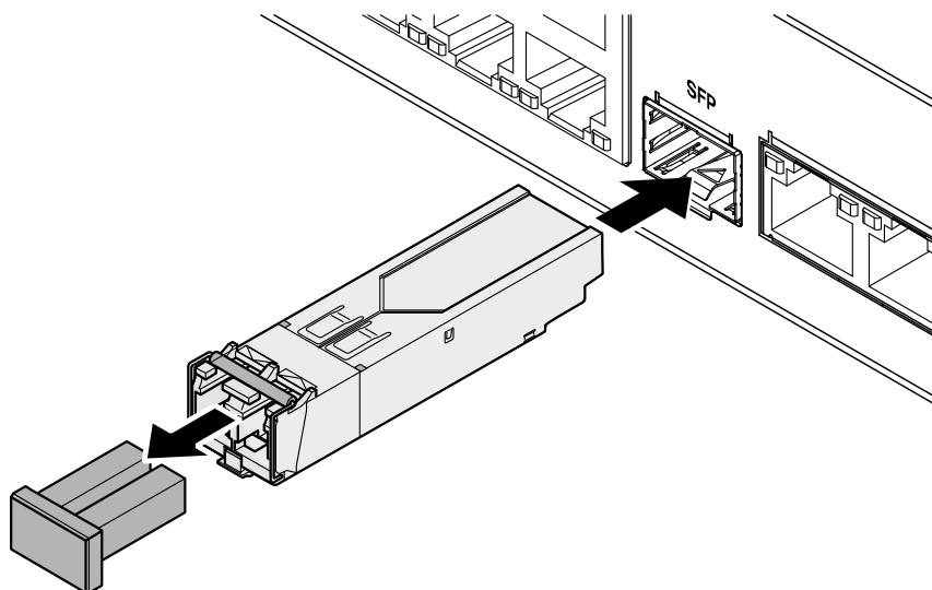
Рисунок 7.1 – Установка SFP-модуля
