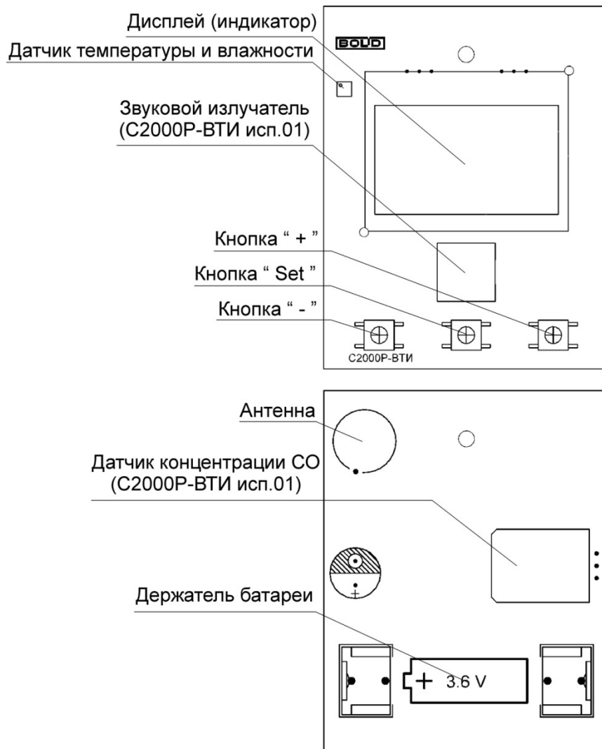
Рисунок 2.3 Расположение элементов на плате
