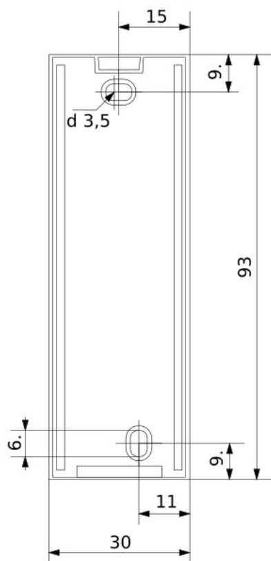
Рисунок 2.3 Монтажные размеры
