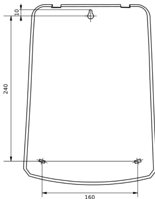
Рисунок 2.3 Монтажные размеры
