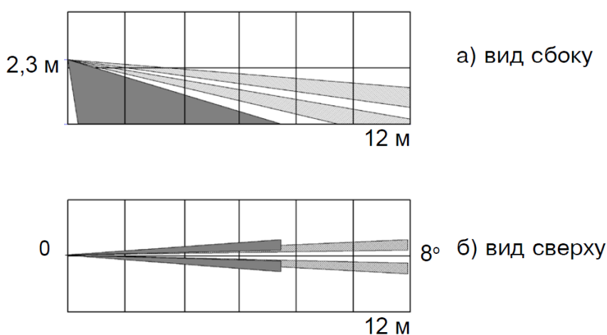
Рисунок 2.5 Зона обнаружения
