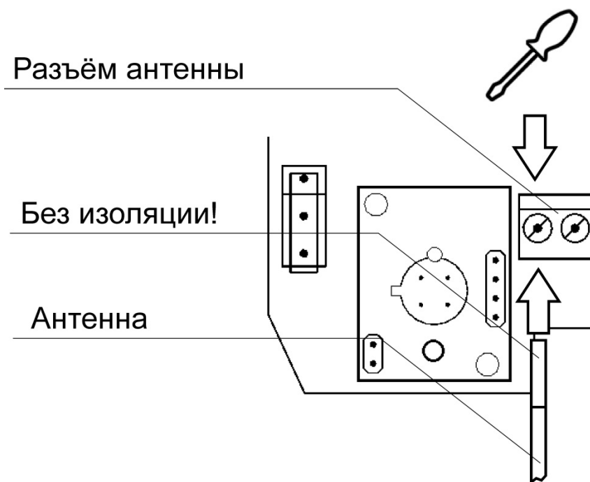
Рисунок 2.4 Установка антенны
