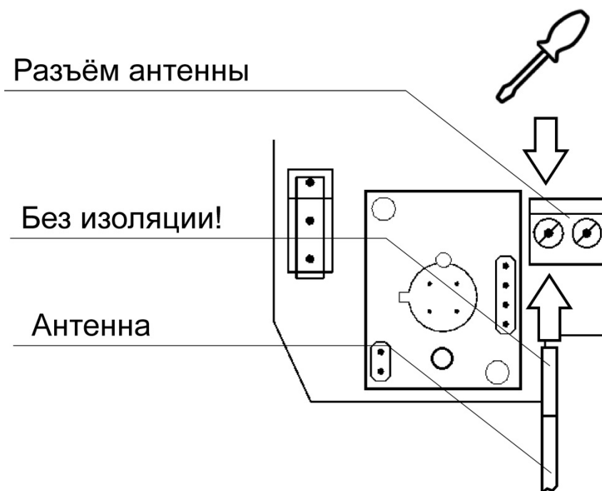
Рисунок 2.4 Установка антенны
