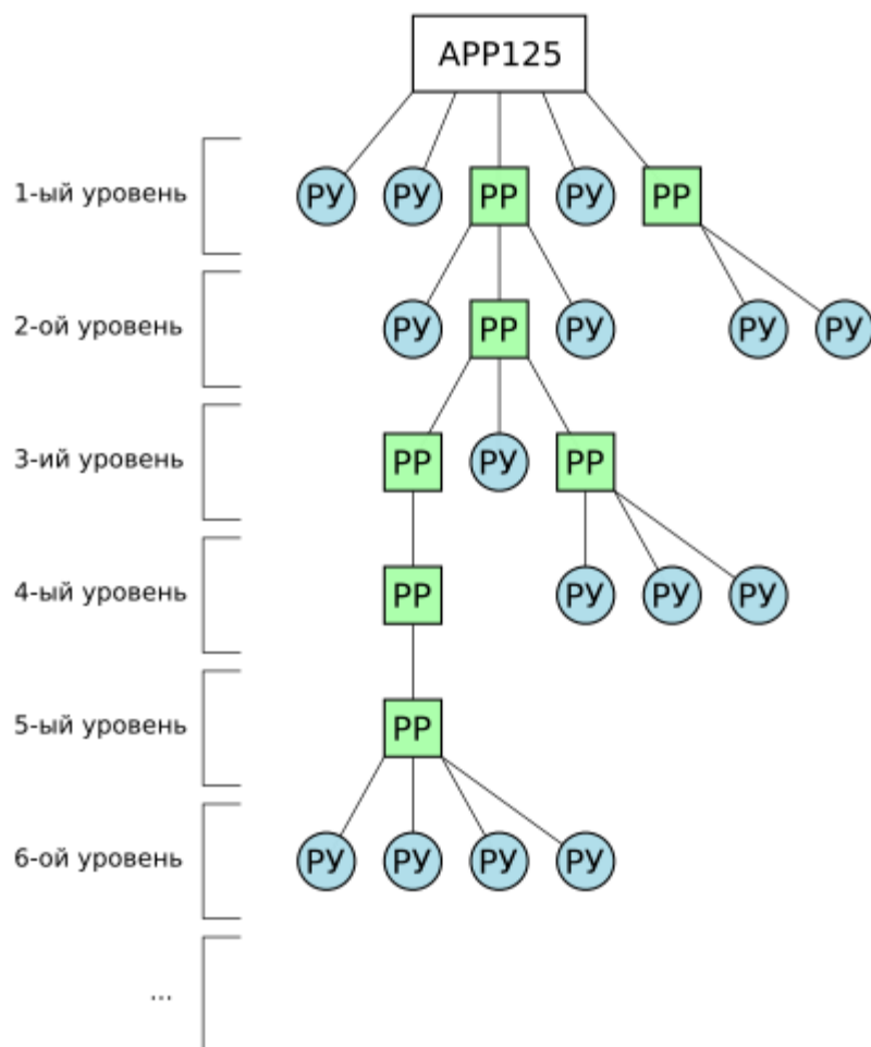
Рисунок 1.4.3-1 Цепь ретрансляции
