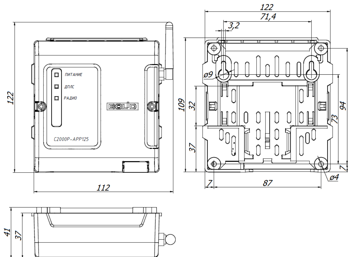
Рисунок 2.2.2.3-2 Габаритные и монтажные размеры C2000P-APP125 апп.14.0
