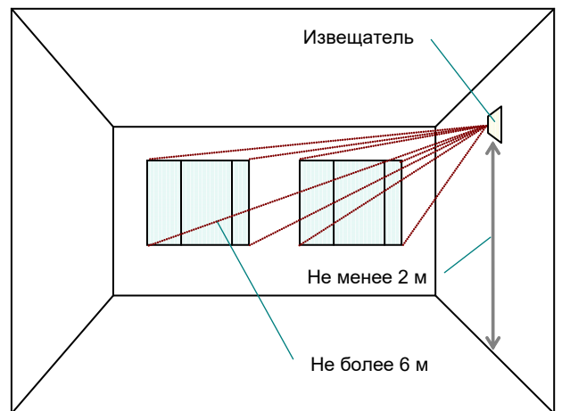
б) установка извещателя на боковой стене
