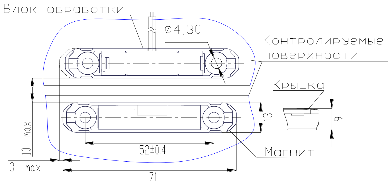
Рисунок 2.2.3.1 Установочные размеры
