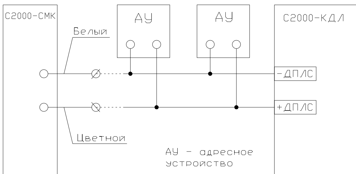
Рисунок 2.2.4.1 Схема подключения
