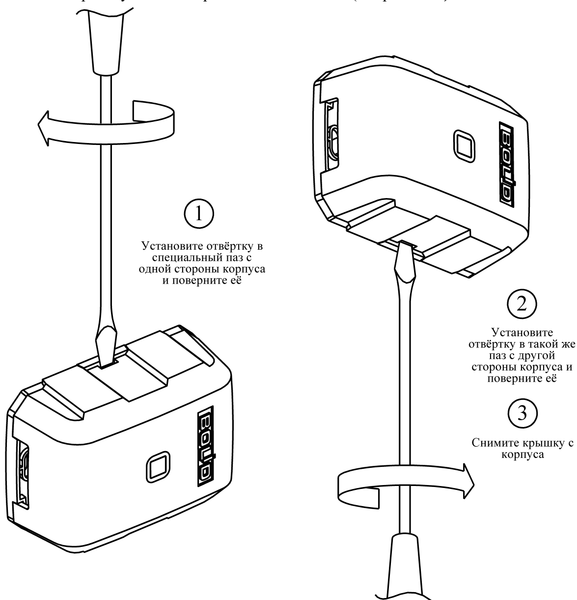
Рисунок 2.2.2 Снятие крышки AP2
