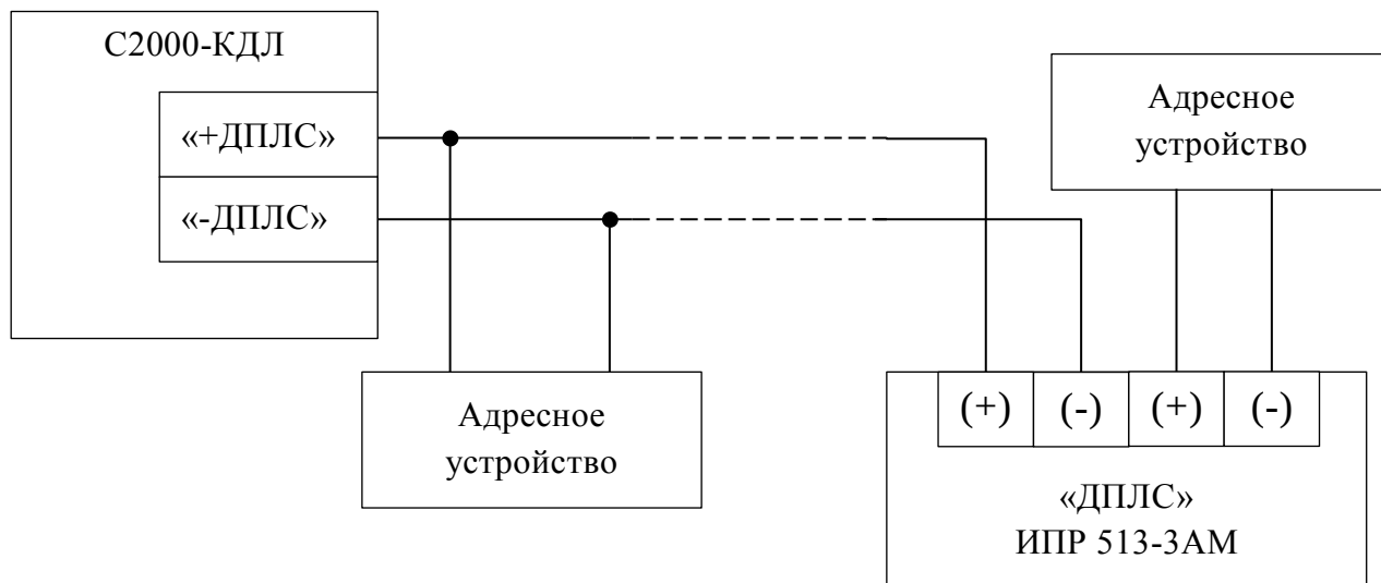
Рисунок 2.2.4.1 Схема внешних соединений
