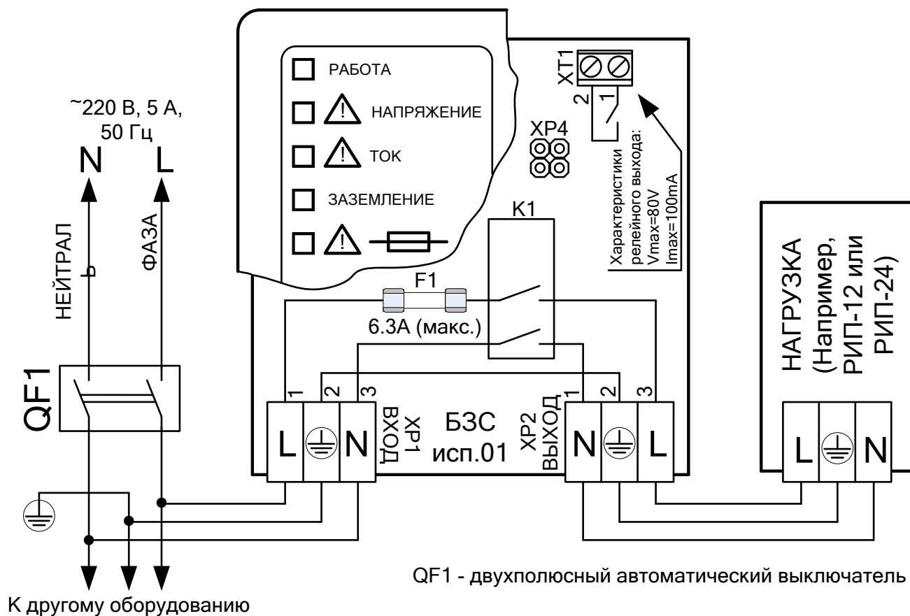
Схема подключения
