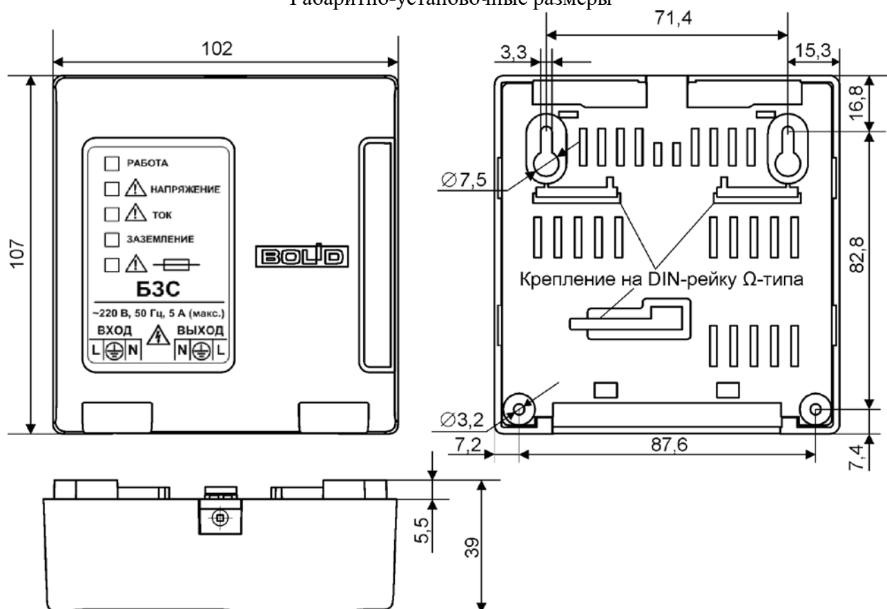
Габаритно-установочные размеры
