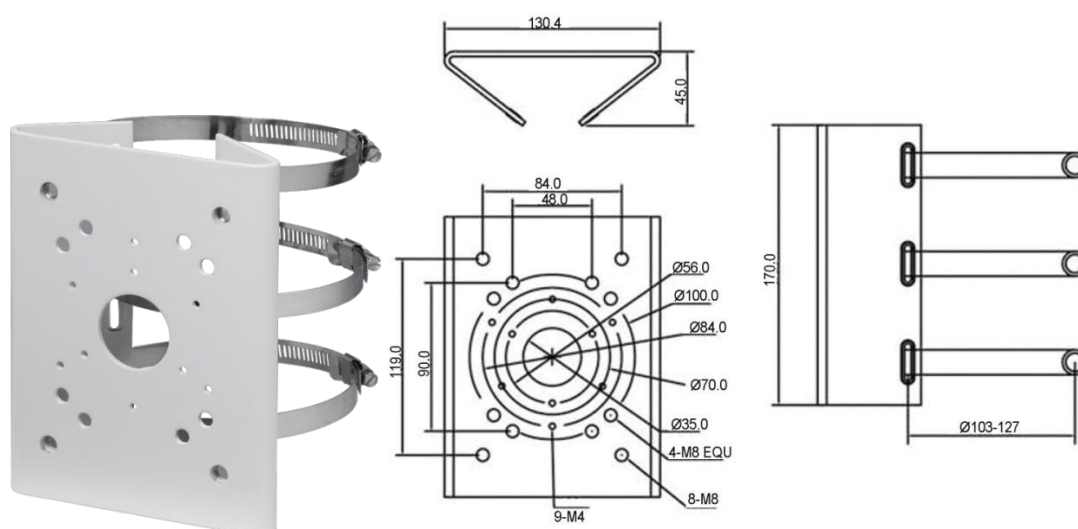
Рисунок 5.10 – Столбовой кронштейн BR-103
