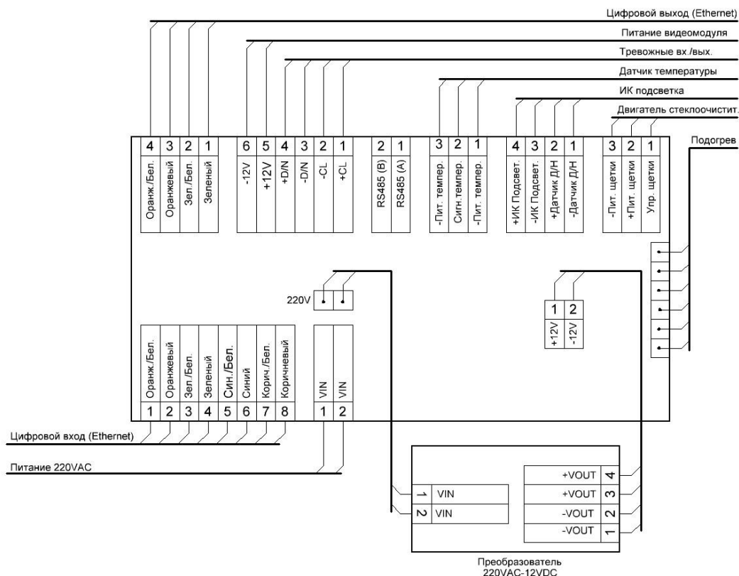
Рисунок 4.6 – Схема подключения термокожуха с напряжением питания 220 В переменного тока
