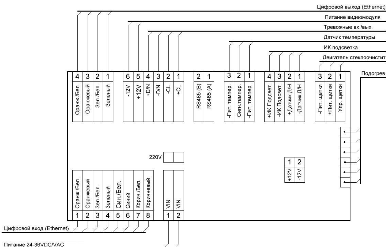
Рисунок 4.7 – Схема подключения термокожуха с напряжением питания 24-36 В постоянного и переменного тока
