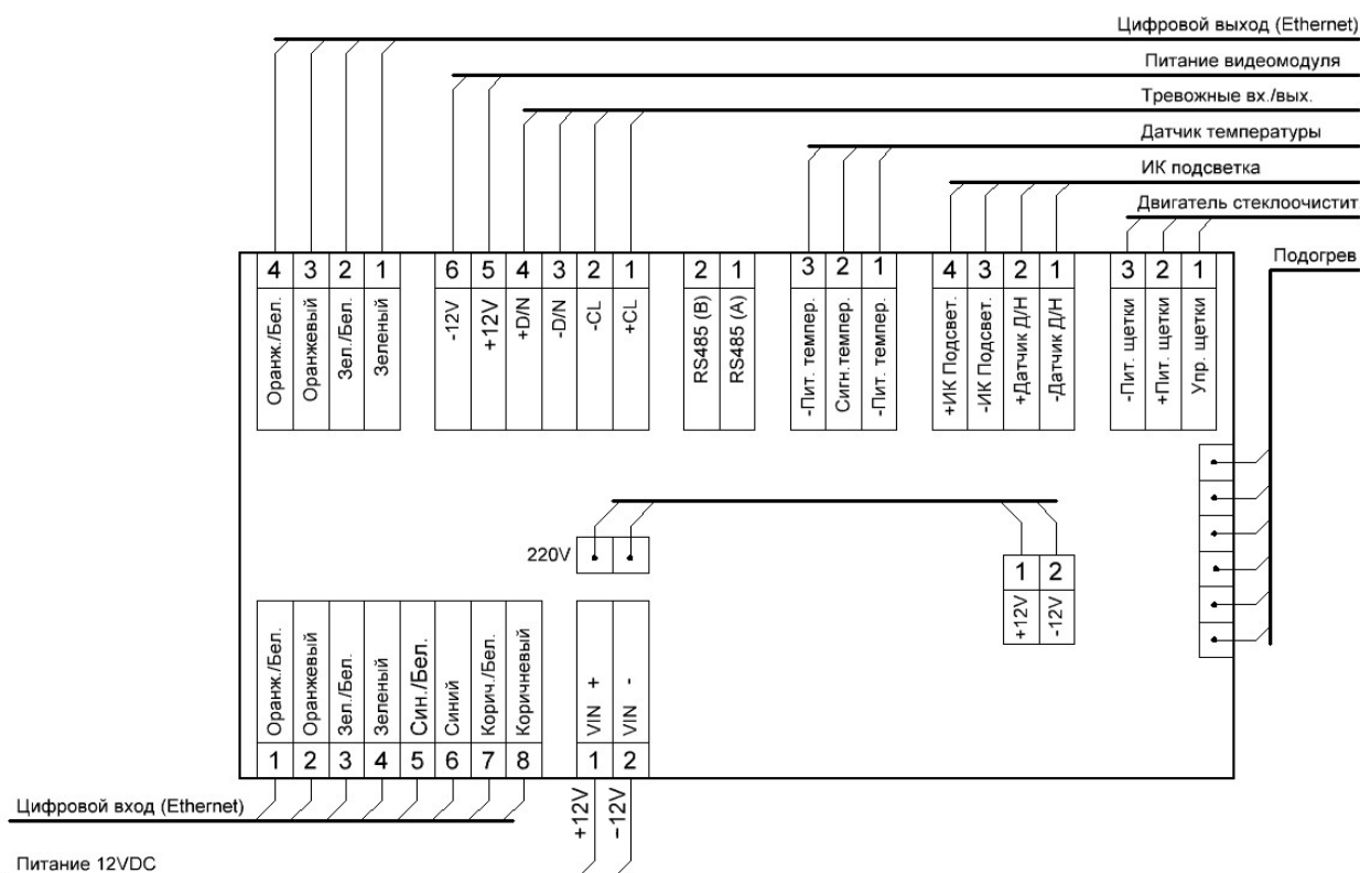
Рисунок 4.5 – Схема подключения термокожуха с напряжением питания 12 В постоянного тока
