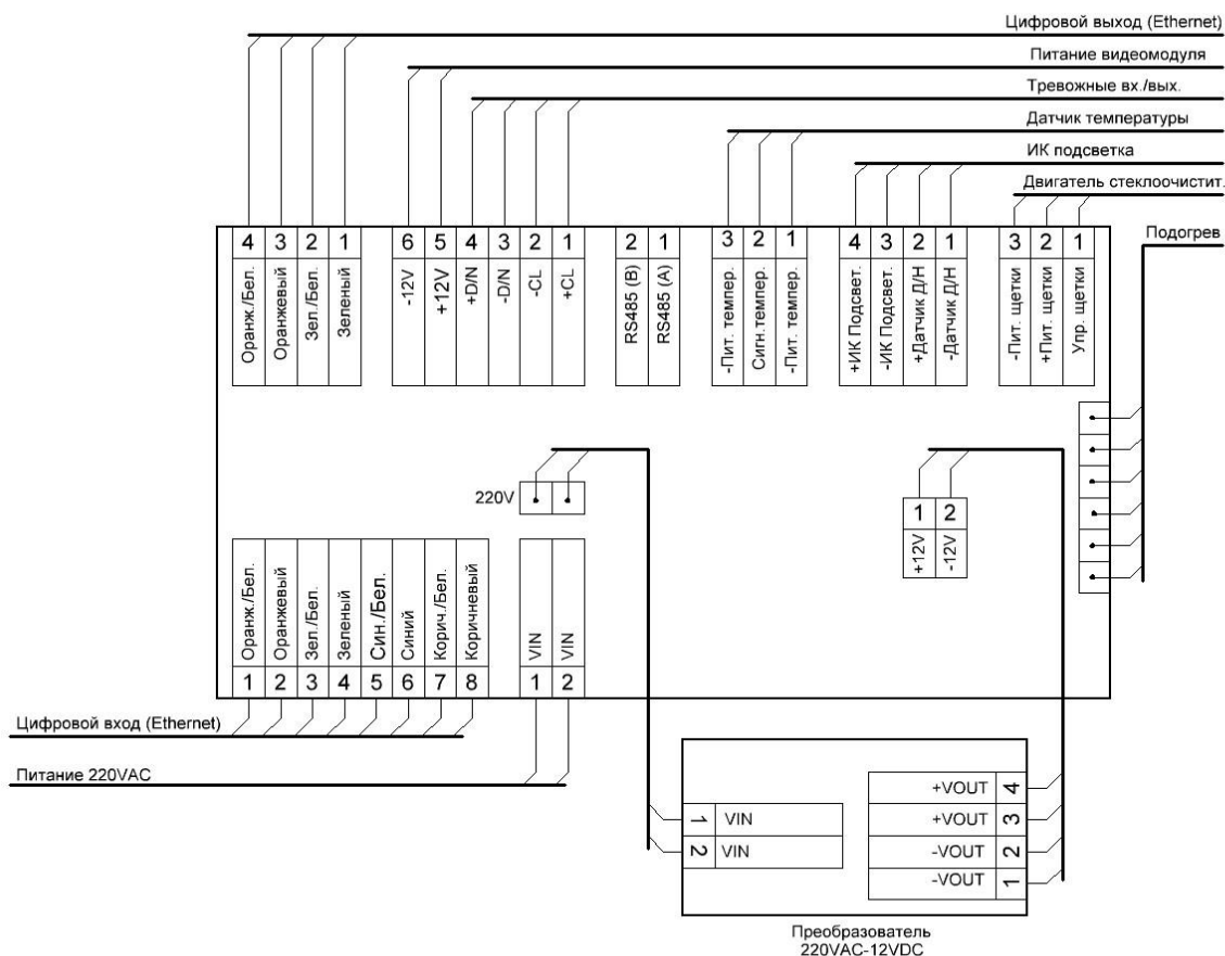
Рисунок 4.3 – Схема подключения термокожуха с напряжением питания 220 В переменного тока
