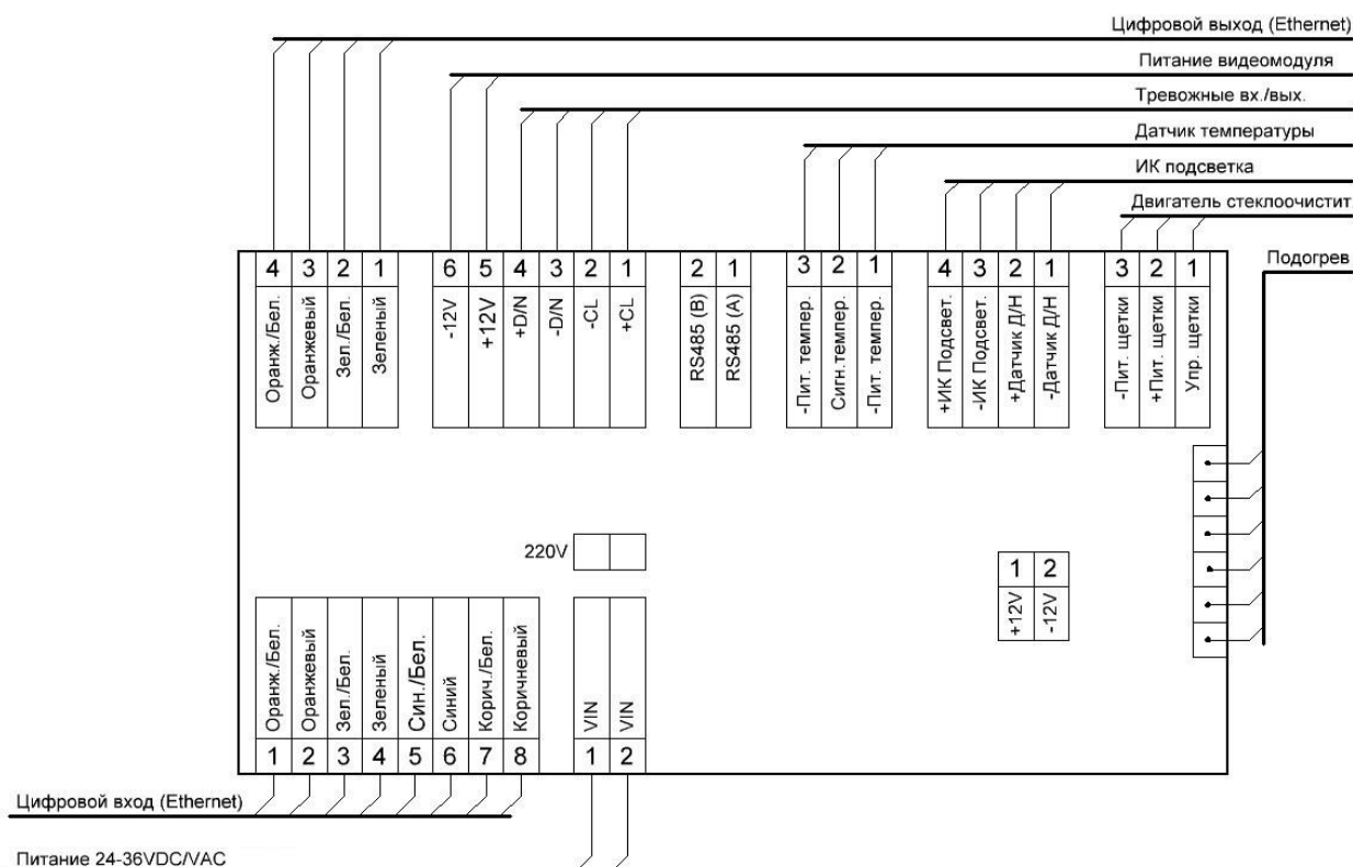
Рисунок 4.4 – Схема подключения термокожуха с напряжением питания 24–36 постоянного и переменного тока
