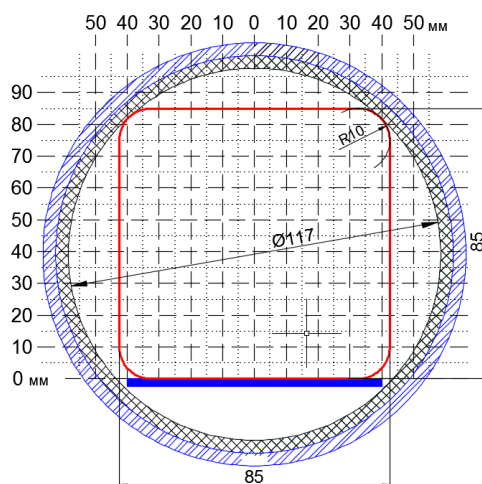
Рисунок 4.3 – Сечение термокожуха
