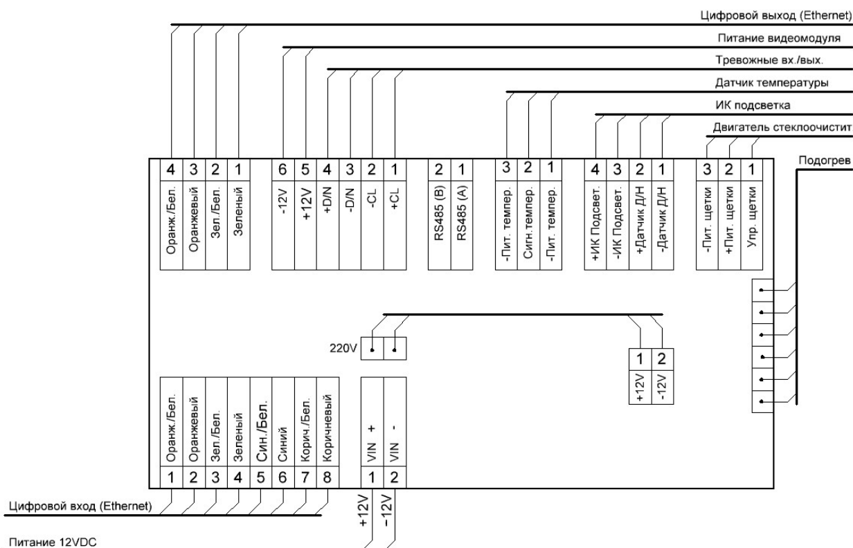
Рисунок 4.8 – Схема подключения термокожуха с напряжением питания 12 В постоянного тока
