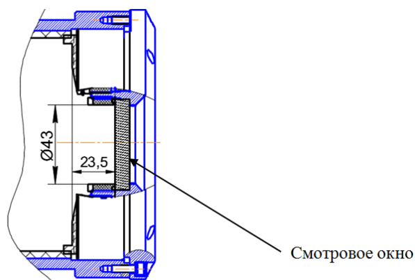
Рисунок 4.2 – Внутреннее пространство смотрового окна
