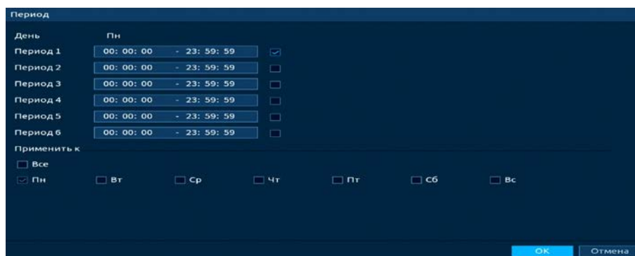
Рисунок 20.48 – Расписание
