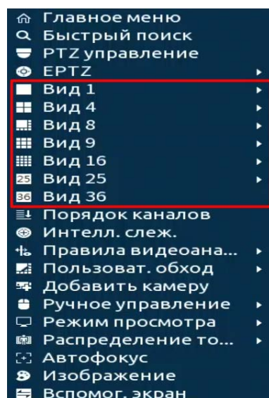
Рисунок 8.1 – Контекстное меню
