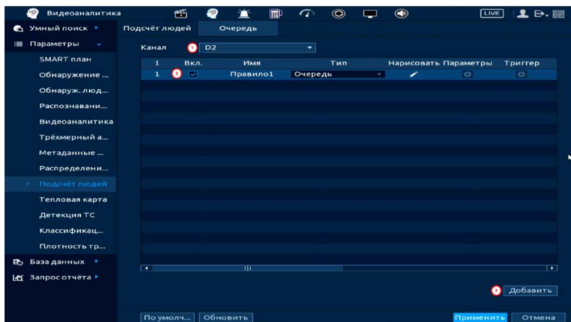
Рисунок 20.112 – Настройка
