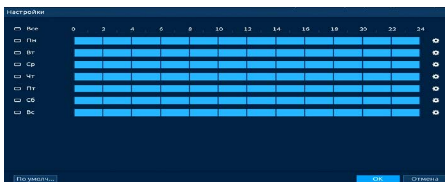
Рисунок 20.125 – Расписание
