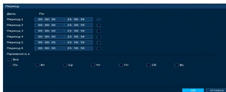
Рисунок 20.24 – Расписание
