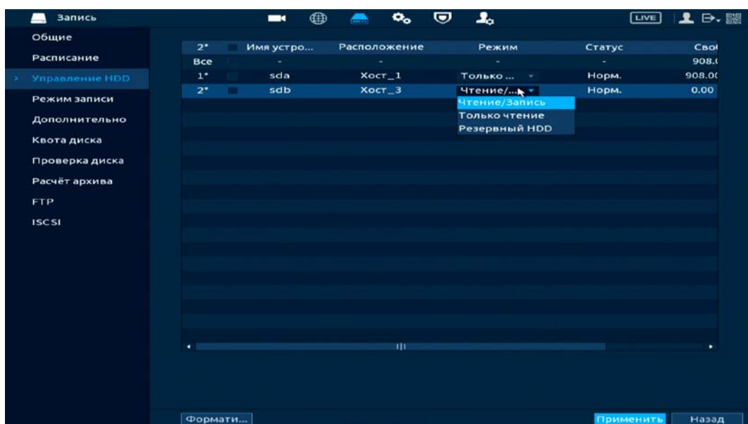
Рисунок 14.15 – Интерфейс настройки
