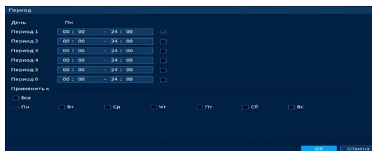
Рисунок 20.92 – Расписание
