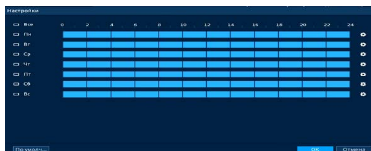
Рисунок 20.91 – Расписание
