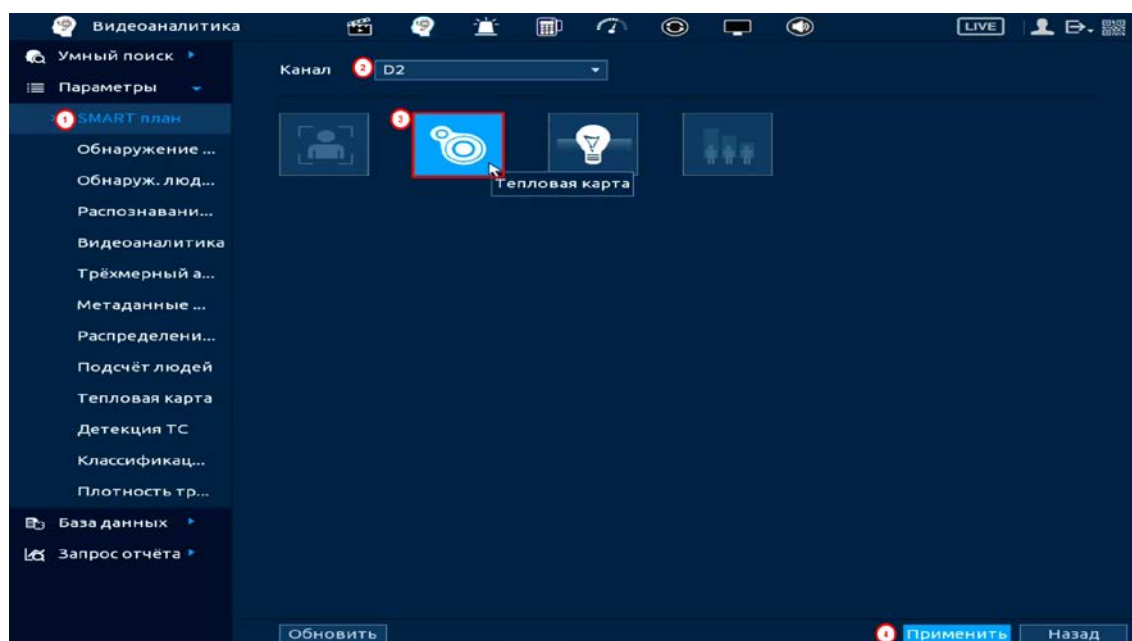
Рисунок 20.119 – Настройка
