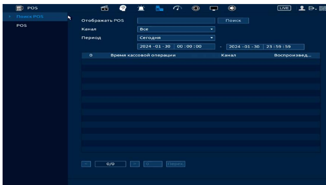
Рисунок 22.1 – POS поиск
