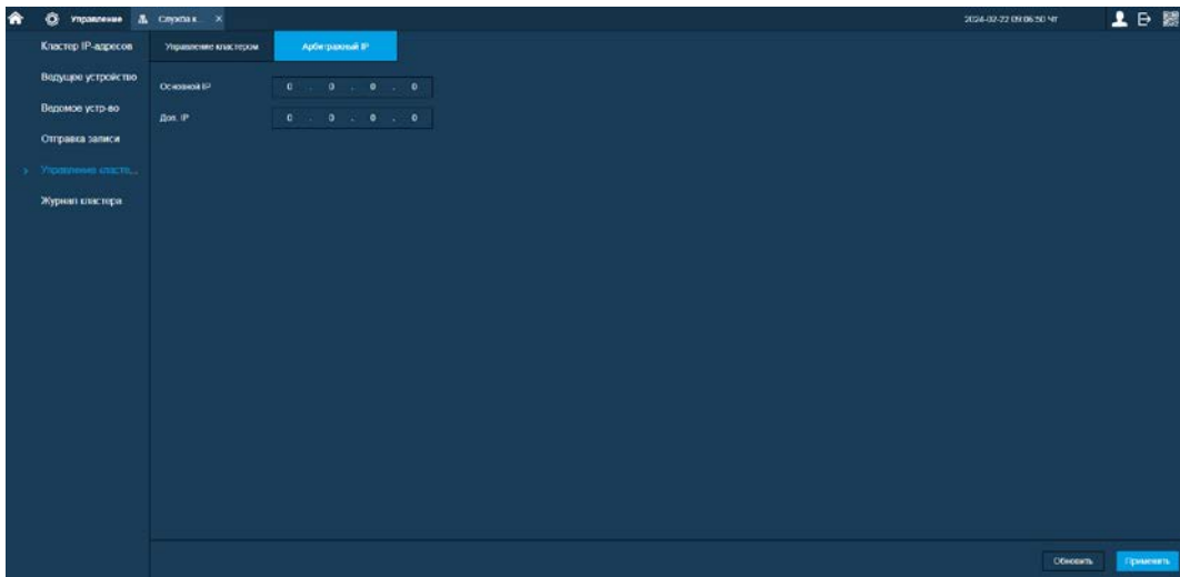
Рисунок 13.33 – Арбитражный IP-адрес
