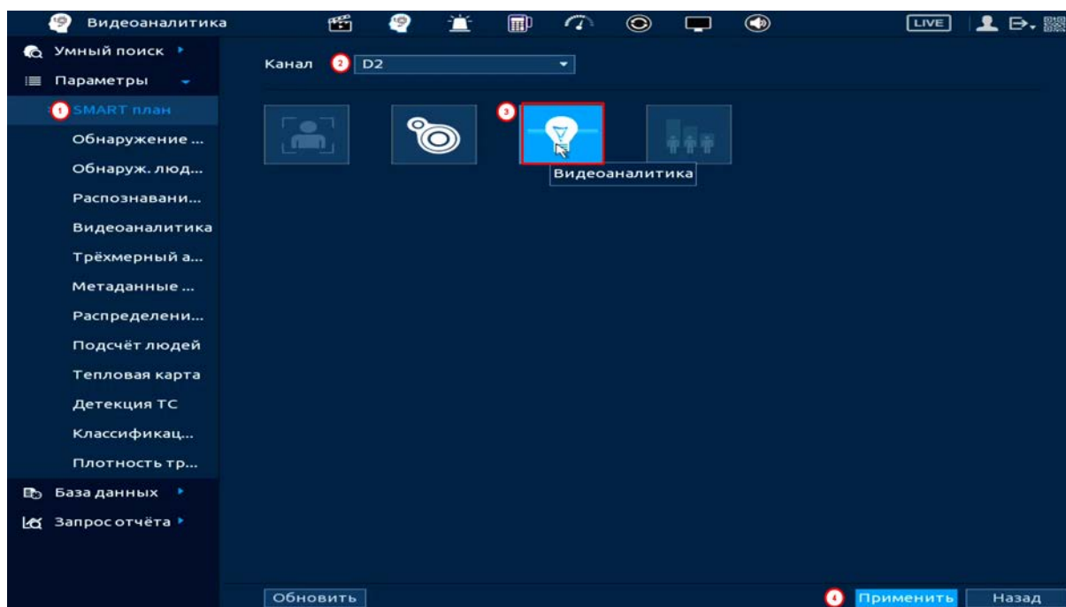
Рисунок 20.49 – Настройка
