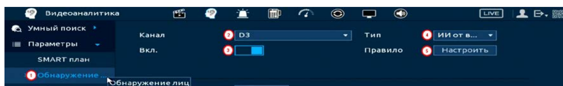
Рисунок 20.15 – Настройка
