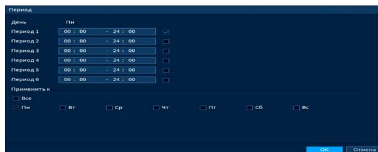
Рисунок 20.72 – Расписание
