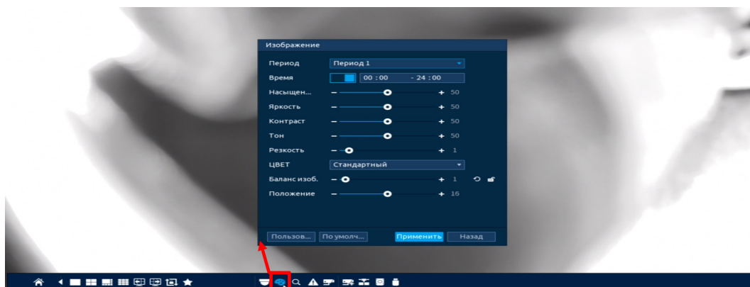
Рисунок 10.2 – Переход в меню редактирования изображения через панель навигации
