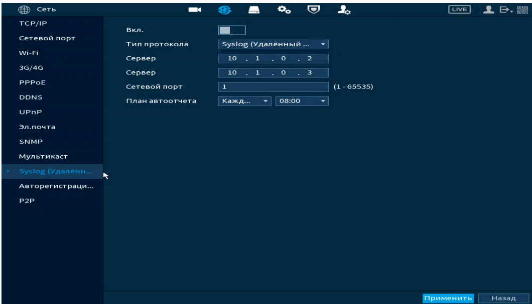
Рисунок 11.13 – Интерфейс настройки «Syslog (Удалённый журнал)»
