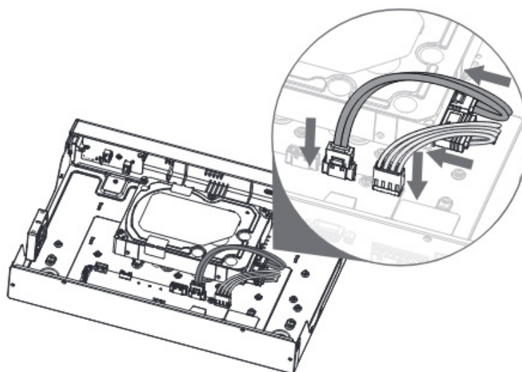
Рисунок 4.7 – Установка жёсткого диска
