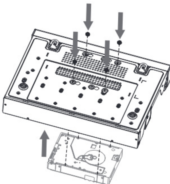
Рисунок 4.6 – Установка жёсткого диска
