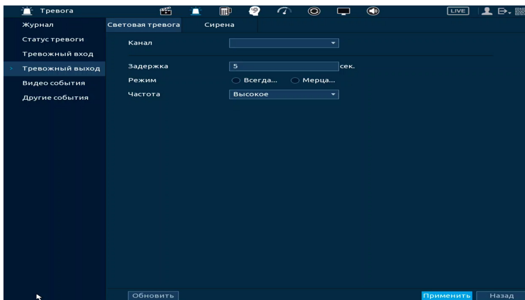
Рисунок 17.14 – Интерфейс настройки «Световая сигнализация»
