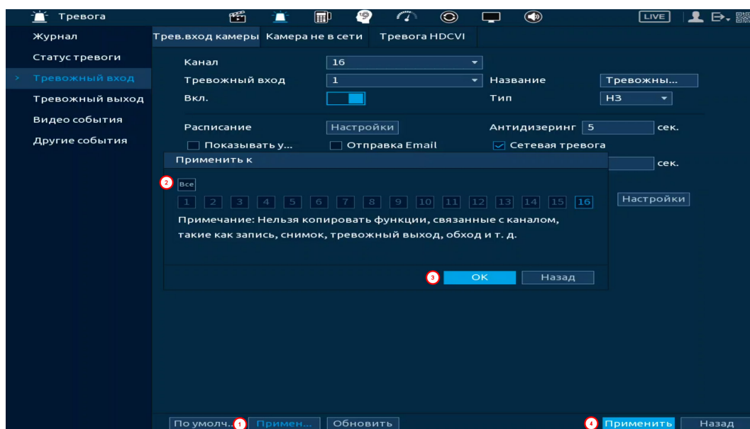
Рисунок 17.6 – Копирование настроек на другие каналы
