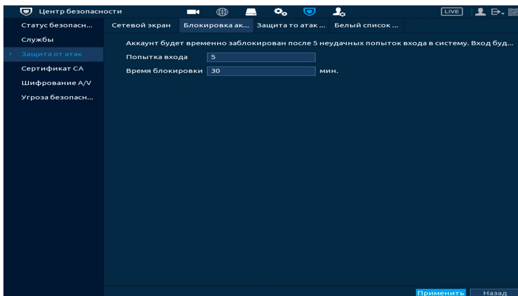
Рисунок 14.12 – Блокировка учётной записи
