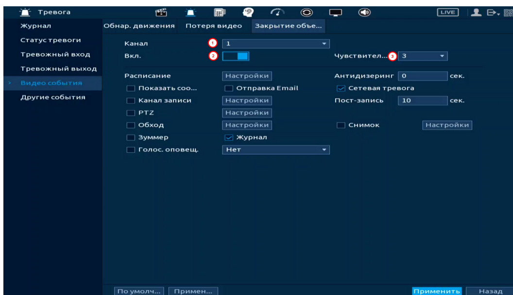
Рисунок 17.25 – Интерфейс настройки закрытия объектива
