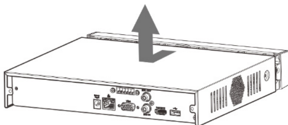
Рисунок 4.4 – Установка жёсткого диска
