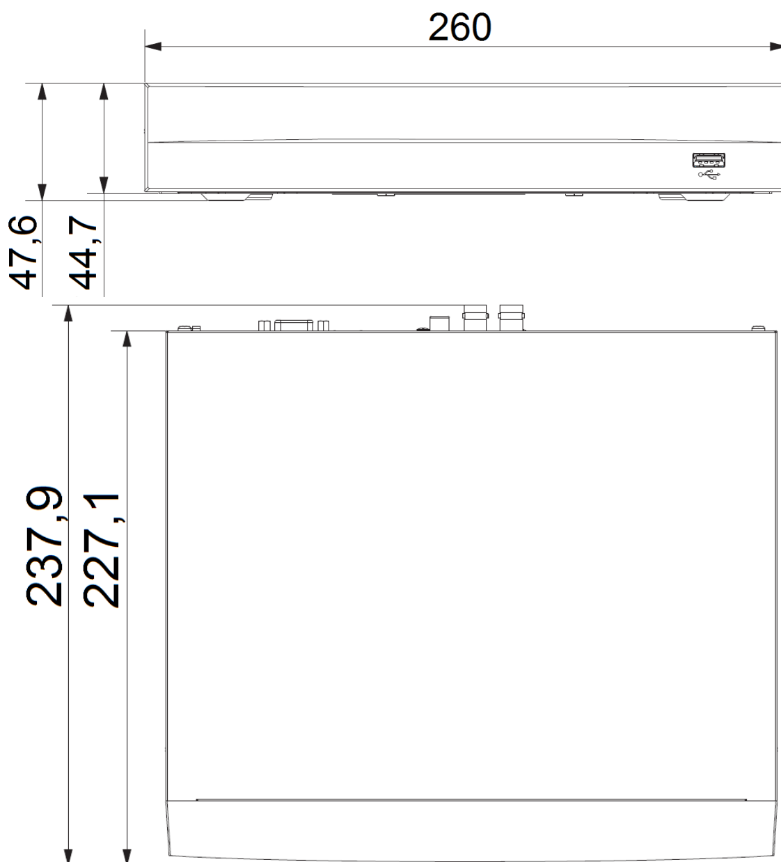
Рисунок 4.2 – Габаритные размеры
