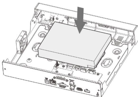
Рисунок 4.5 – Установка жёсткого диска
