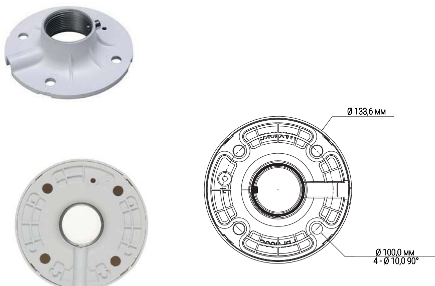
Рисунок 4.2 – Монтажное основание кронштейна BR-104
