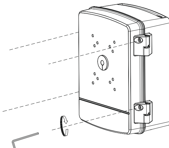
Рисунок 4.4 – Монтаж
