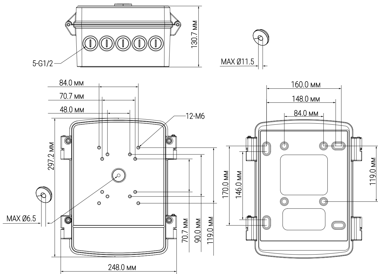
Рисунок 4.1 – Габаритные размеры
