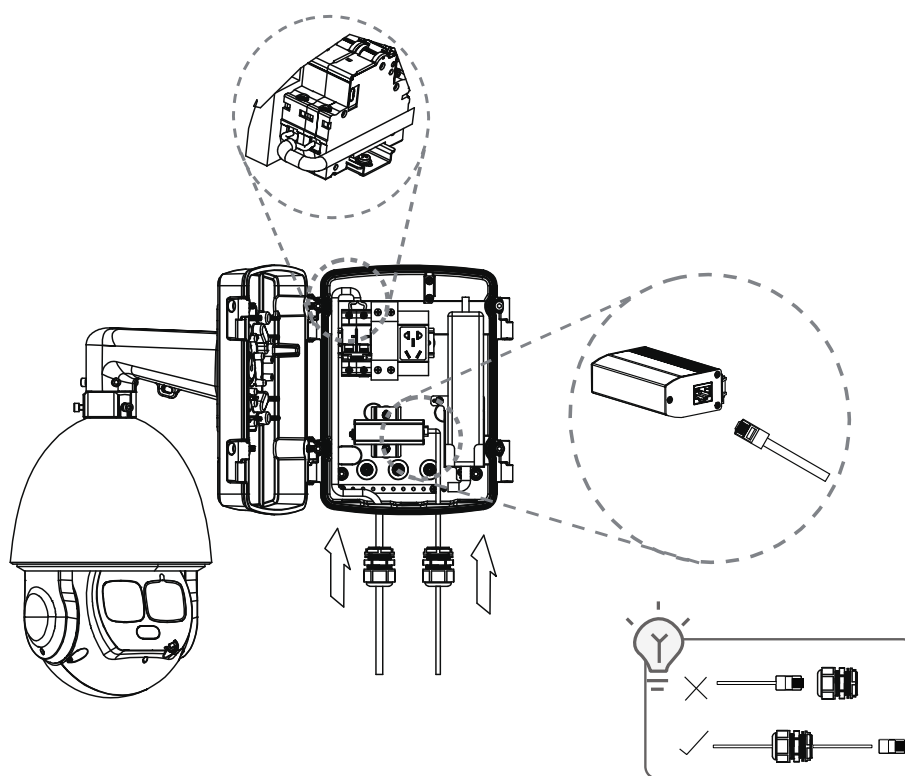
Рисунок 4.10 – Монтаж
