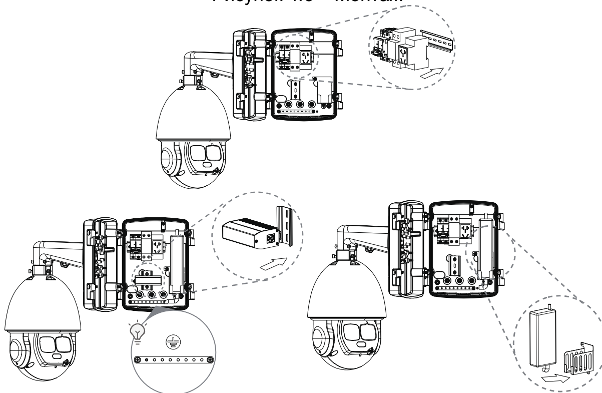
Рисунок 4.7 – Монтаж
