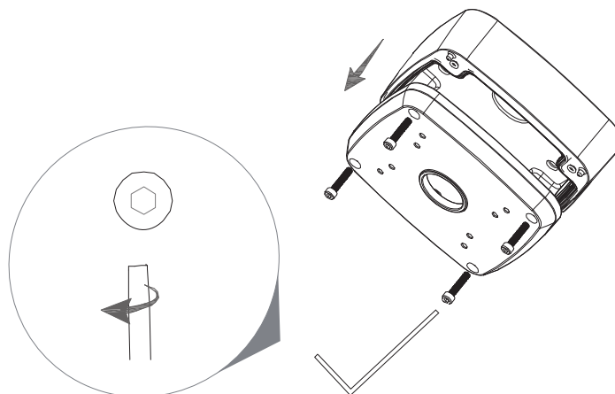
Рисунок 4.2 – Монтаж
