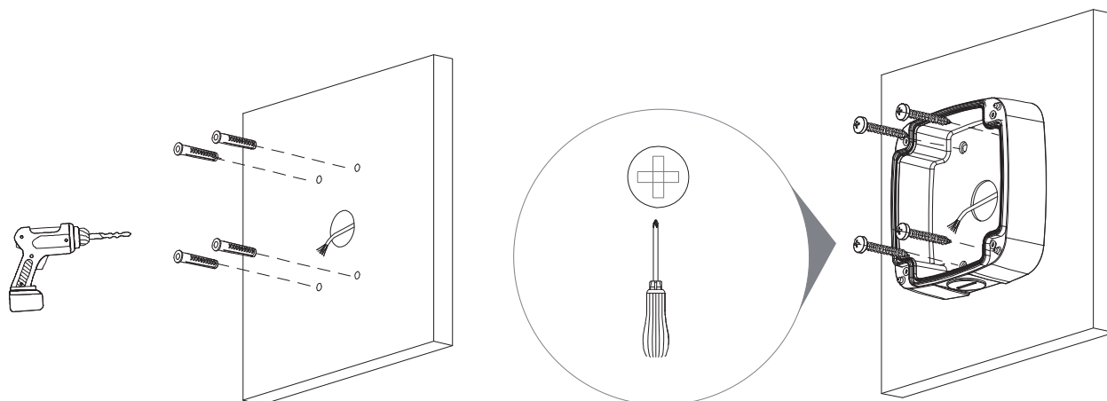
Рисунок 4.3 – Монтаж
