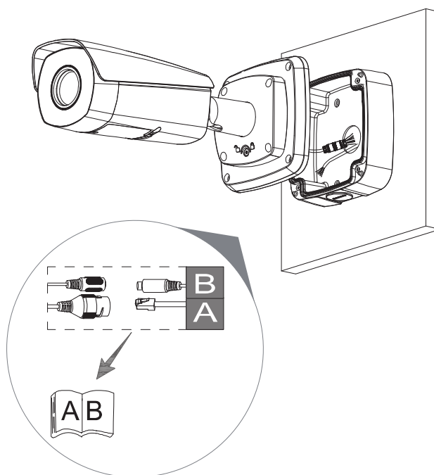
Рисунок 4.5 – Монтаж
