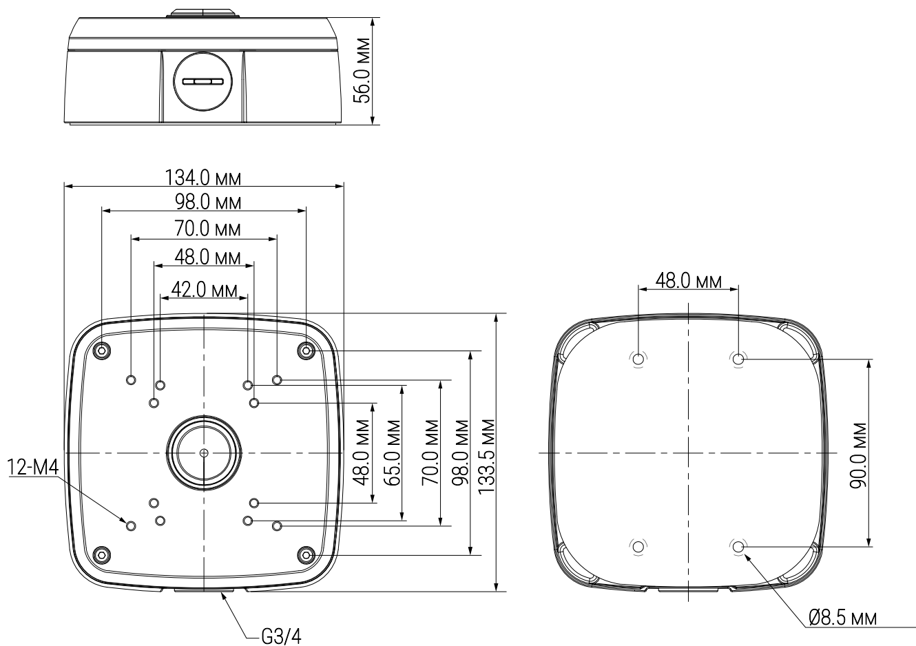
Рисунок 4.1 – Габаритные размеры
