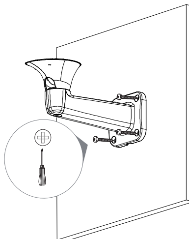
Рисунок 4.3 – Монтаж
