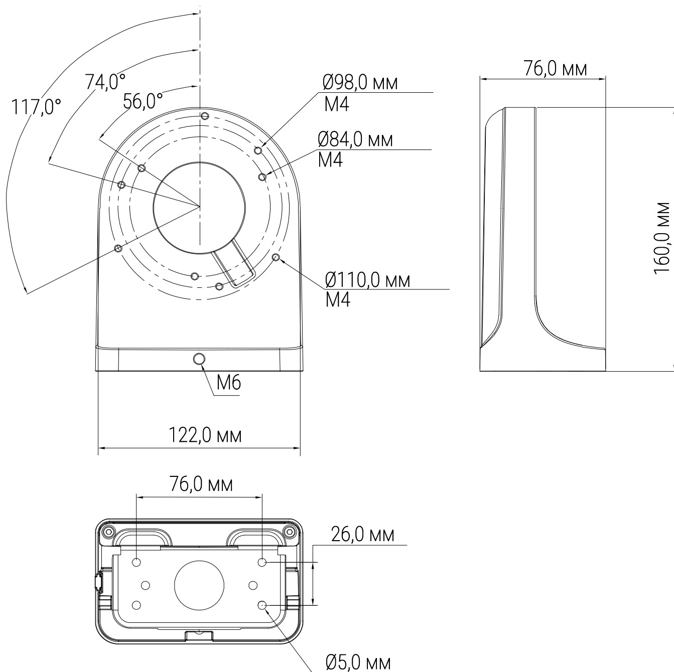
Рисунок 4.1 – Габаритные размеры
