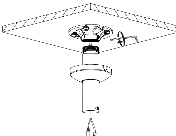
Рисунок 5.4 – Монтаж
